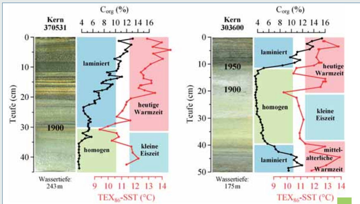
ABB. 1: ZWEI KURZKERNE AUS UNTERSCHIEDLICHEN WASSERTIEFEN IM GOTLANDBECKEN. SCHWARZE KURVE: ORGANISCHER KOHLENSTOFFGEHALT (C ORG ). ROTE KURVE: REKONSTRUKTION VON OBERFLÄCHENWASSERTEMPERATUREN MIT HILFE DES BIOMARKERS TEX86 (TEX86-SST). LAMINIERT UND HOMOGENE BEREICHE SOWIE DIE ZEITLICHE EINTEILUNG IN MITTELALTERLICHE WARMZEIT, KLEINE EISZEIT UND HEUTIGE WARMZEIT SIND GEKENNZEICHNET, EBENSOWIE DIE ZEITPUNKTE DES ÜBERGANGS VON OXISCHEN (HOMOGEN) ZU ANOXISCHEN (LAMINIERT) BEDINGUNGEN. / TWO SHORT SEDIMENT CORES FROM DIFFERENT WATER DEPTHS OF THE GOTLAND BASIN. BLACK CURVE: ORGANIC CARBON (C ORG ). RED CURVE: RECONSTRUCTION OF SEA SURFACE TEMPERATURES BY MEANS OF THE BIOMARKER TEX86.
