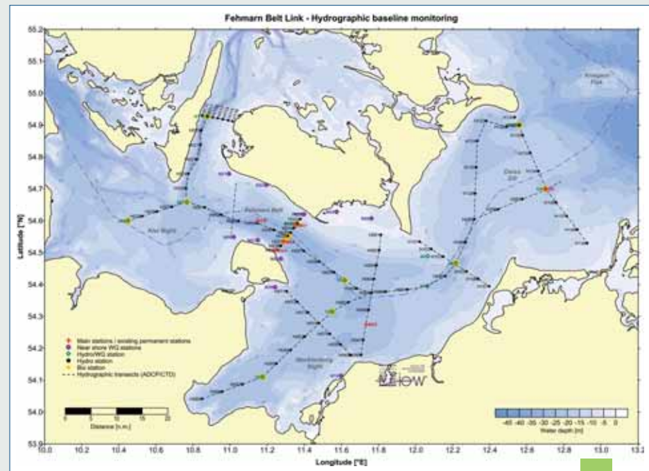
ABB. 1: DAS STATIONSNETZ DES MONITORING-PROGRAMMES IM SEEGEBIET UM DEN FEHMARNBELT. DIE ROTEN PUNKTE KENNZEICHNEN DIE VERANKERTEN HAUPTSTATIONEN, DIE LILA PUNKTE DIE TRÜBUNGSMESSSTATIONEN. DIE GESTRICHELTEN LINIEN ZEIGEN DIE OZEANOGRAPHISCHEN SCHNITTE MIT DEN CTD STATIONEN. / THE POSITION OF THE MOORED STATIONS AND TRANSECTS WORKED IN THE FEHMARNBELT AREAS. RED DOTS INDICATE MOORED MAIN STATIONS, VIOLET DOTS THE STATIONS MEASURING TURBIDITY. DASHED LINES SHOW THE OCEANOGRAPHIC TRANSECTS WITH THE CTD STATIONS.
