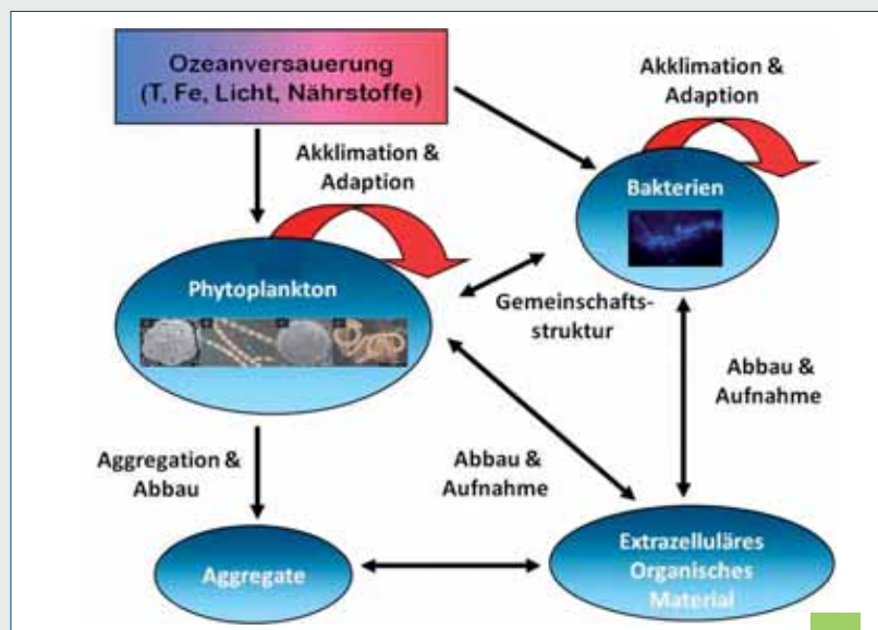
ABB. 1: SCHEMA ZUM EINFLUSS DER OZEANVERSÄUERUNG AUF VERSCHIEDENE EBENEN DES NÄHRUNGSNETZES (PHYTOPLANKTON, BAKTERIEN) UND DEREN GEGENSEITIGE BEEINFLUSSUNG SOWIE DER EINFLUSS AUF STOFFKREISLÄUFE (AGGREGATION, PRODUKTION UND ABBAU VON GELÖSTEM ORGANISCHEM MATERIAL). / THE IMPACT OF OCEAN ACIDIFICATION ON THE DIFFERENT LEVELS OF THE FOOD WEB (PHYTOPLANKTON, BACTERIA), THEIR INTERRELATIONS AND THE MATTER FLUXES (AGGREGATION, PRODUCTION AND DECOMPOSITION OF DISSOLVED ORGANIC MATTER)
